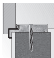
Kampinio profilio - LARGE durų staktos montavimas su kaišiais
