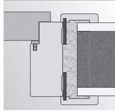
Montavimas betono sienoje su montavimo putomis
