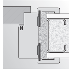
montavimas gipso kartono sienoje su putomis
