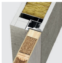
Durų varčia be užlaidos (išorinis varstymas) dešininės
