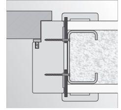
montavimas gipso kartono sienoje su varžtais
