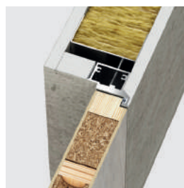
Durų varčia su atvirkštine užlaida (vidinis varstymas) kairinės
