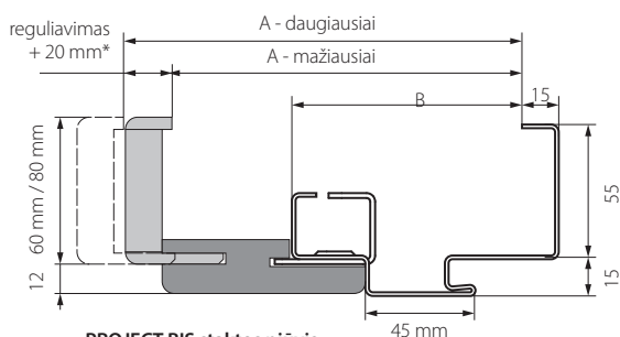
PROJECT BIS staktos pjūvis
