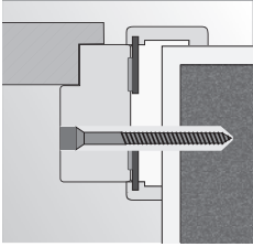
Montavimas betono sienoje naudojant montavimo putas ir ankerius
