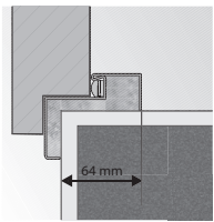
Kampinio profilio durų stakta - SMALL PLUS
