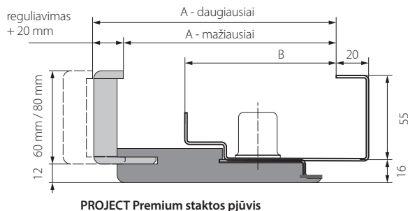
PROJECT Premium staktos pjūvis
