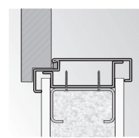
Kampinio profilio - LARGE durų staktos montavimas gipso kartono sienoje
